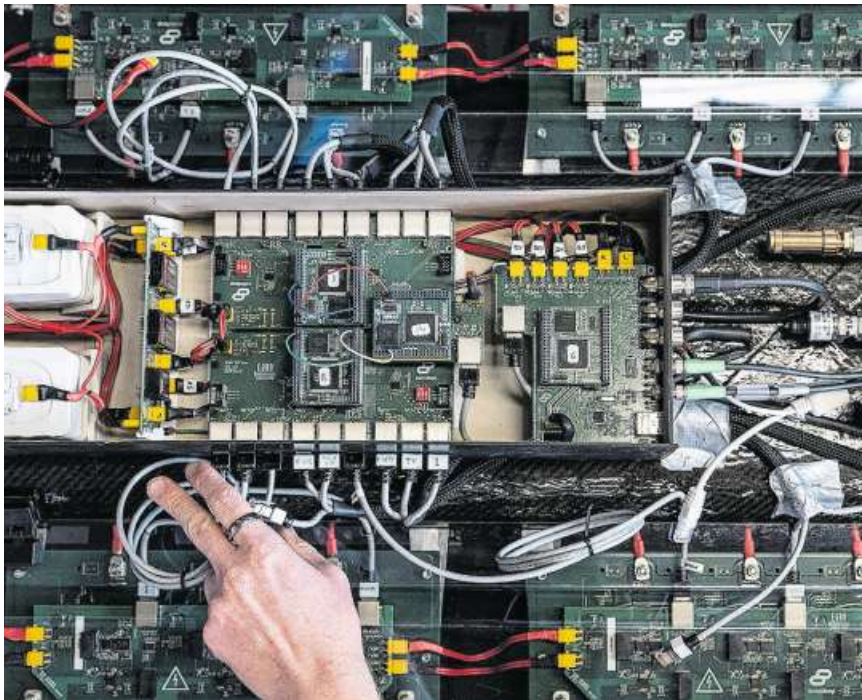
1741 Einzelteile finden sich unter der Swissloop-Haube.
